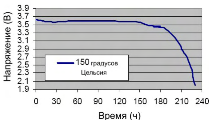
График разряда батареи при высокой температуре 100 мА
