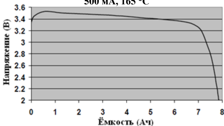
График разряда батареи при высокой температуре 500 мА, 165 °С
