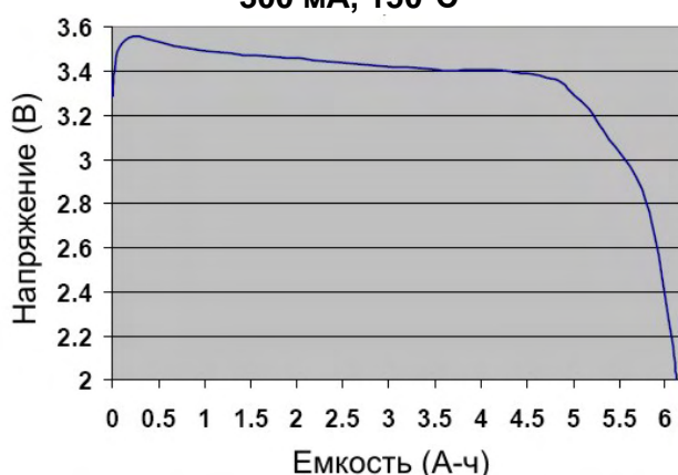
График разряда батареи при высокой температуре 300 мА, 150°C
