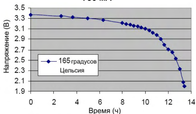
График разряда батареи при высокой температуре 750 мА
