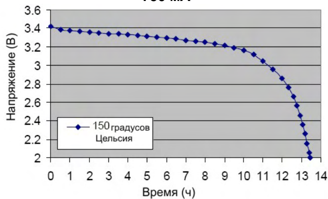
График разряда батареи при высокой температуре 750 мА
