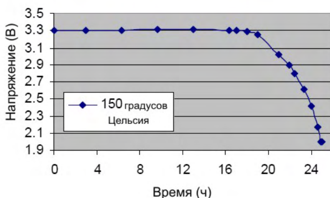
График разряда батареи при высокой температуре 750 мА
