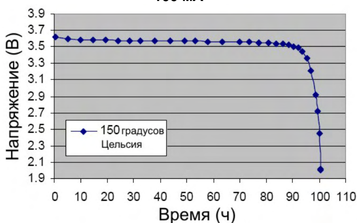
График разряда батареи при высокой температуре 100 мА
