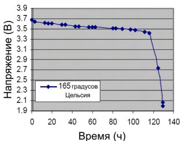
График разряда батареи при высокой температуре 50 мА
